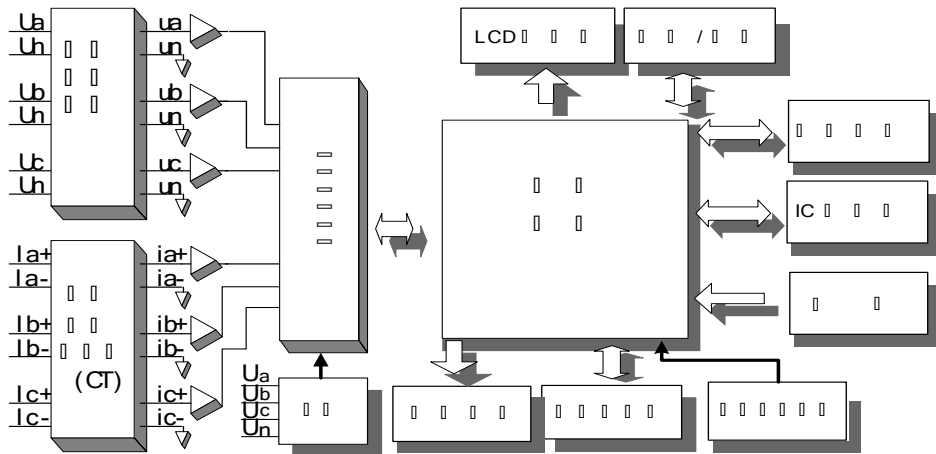
图 1：工作原理简述（以三相四线表为例）
