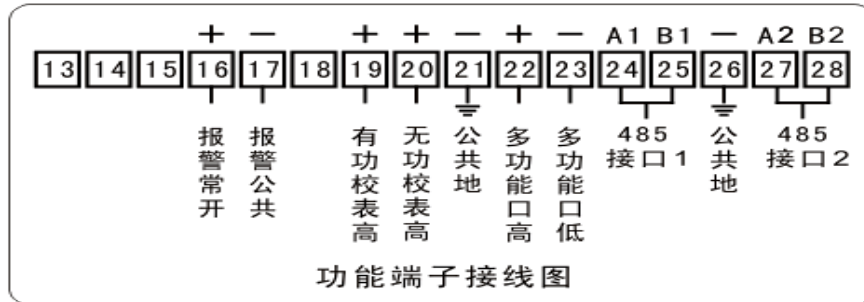
图 7：辅助端子排列图
